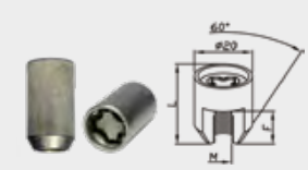
NUT 60° DADO 60°
