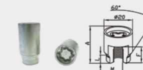
CONICAL NUT + CYLINDRICAL 60° DADO CONICO + CILINDRICO 60°
