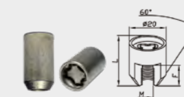
NUT 60° DADO 60°
